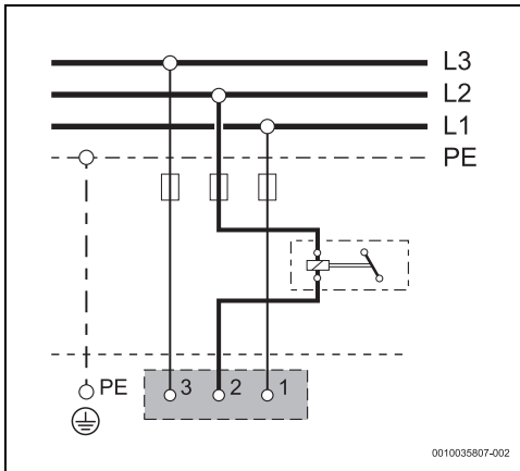
Bild 41 Schaltplan
