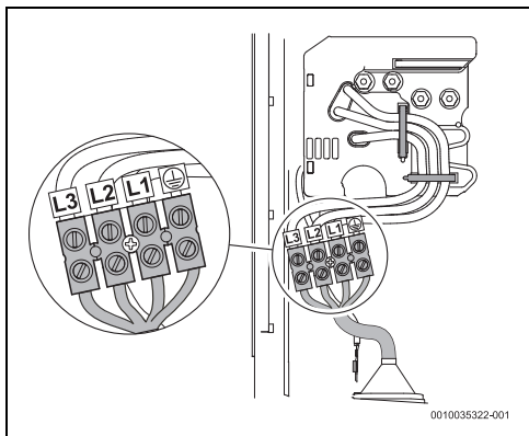
Bild 43 Anschluss unten
