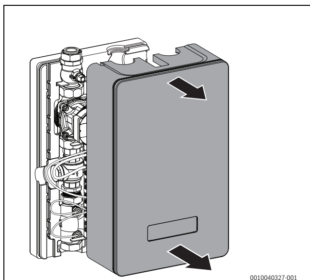
Bild 5 Vorderen Wärmeschutz abnehmen
