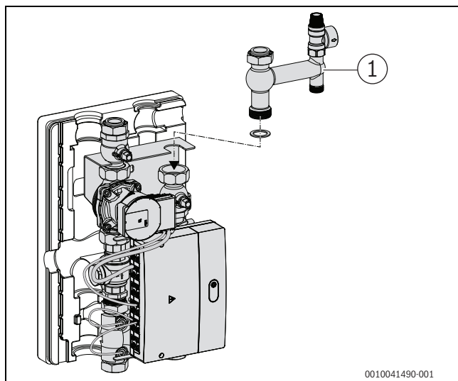
Bild 6 Sicherheitsventil montieren
