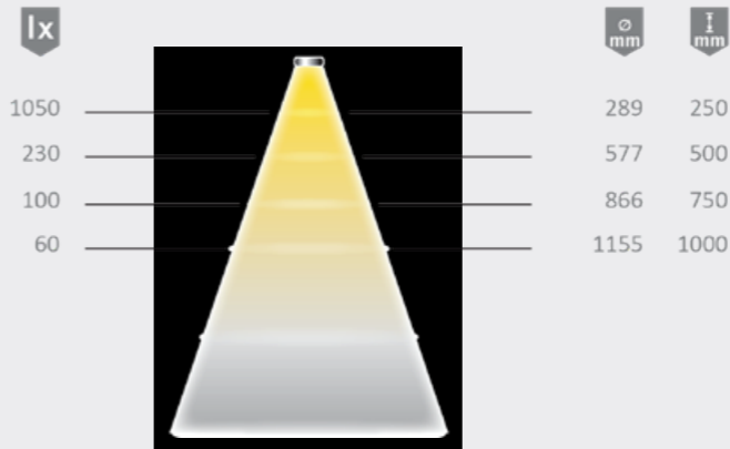
Lichtverteilungsdiagramm 60° - im schwarzen Raum gemessen
