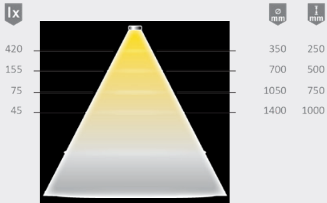
Lichtverteilungsdiagramm 70° - im schwarzen Raum gemessen
