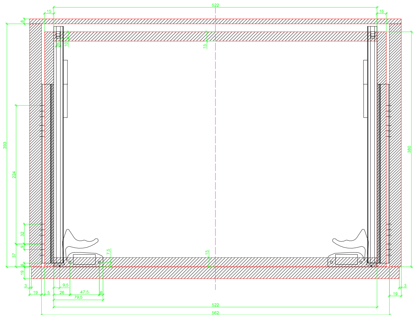
Grooved drawer slide without Plug/ Genutete Seitenzarge ohne Aufsteckhalter
