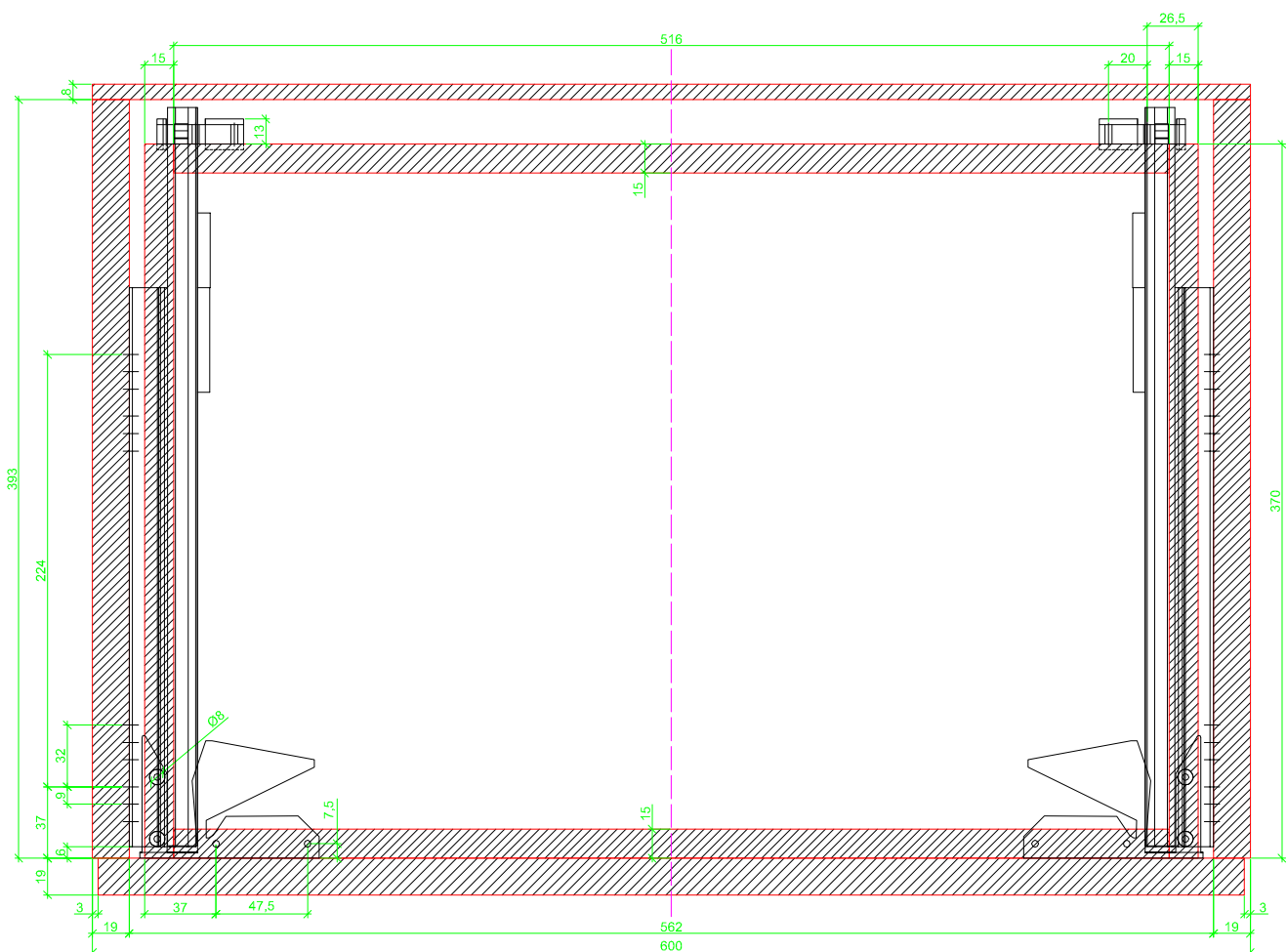
Drawer slide on top of drawer bottom with Plug/ Seitenzarge auf Schubkastenboden mit Aufsteckhalter
