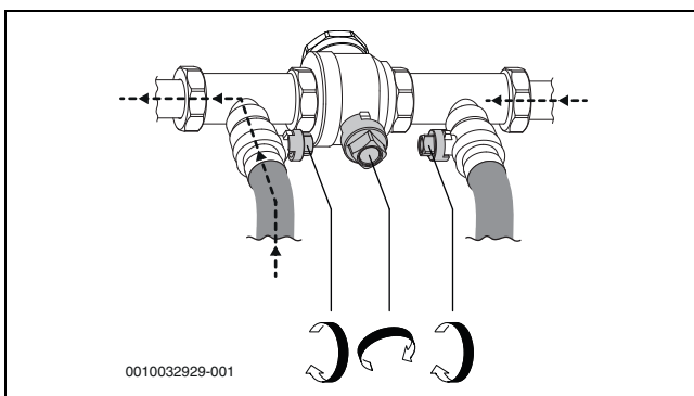
Bild 32 Befülleinrichtung in Druckerhöhungsposition
