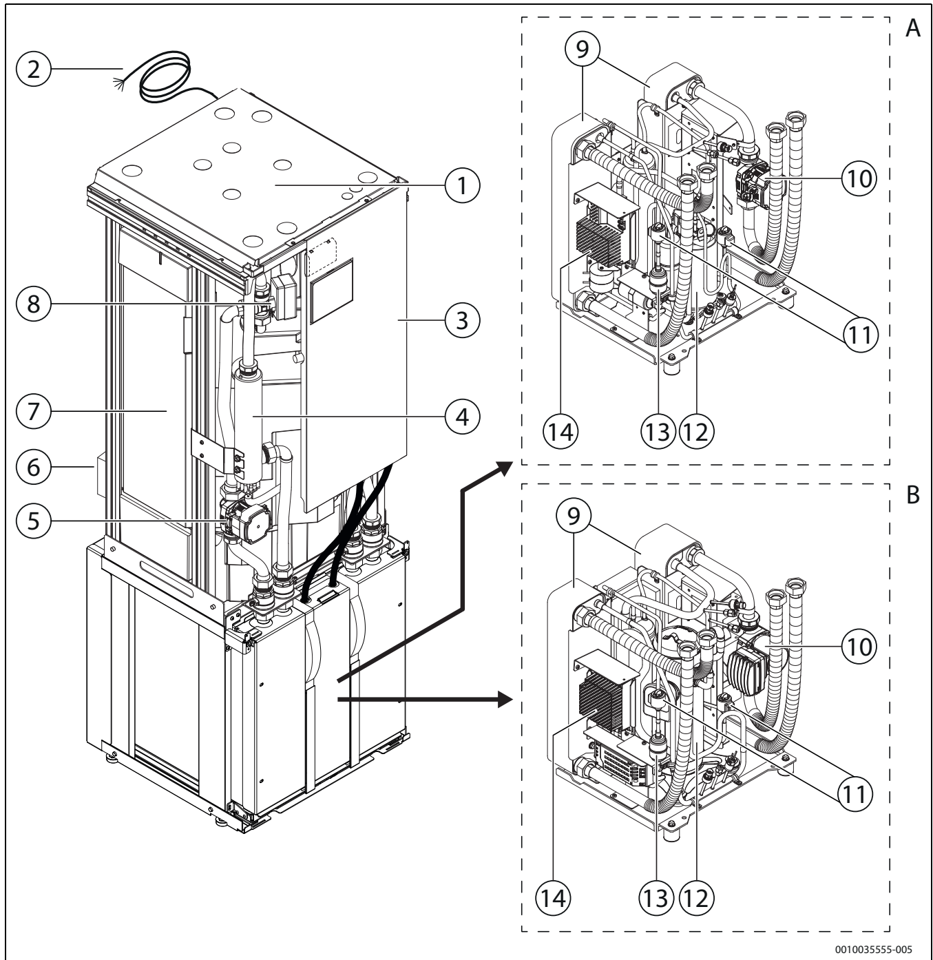
Bild 3 Produktübersicht
