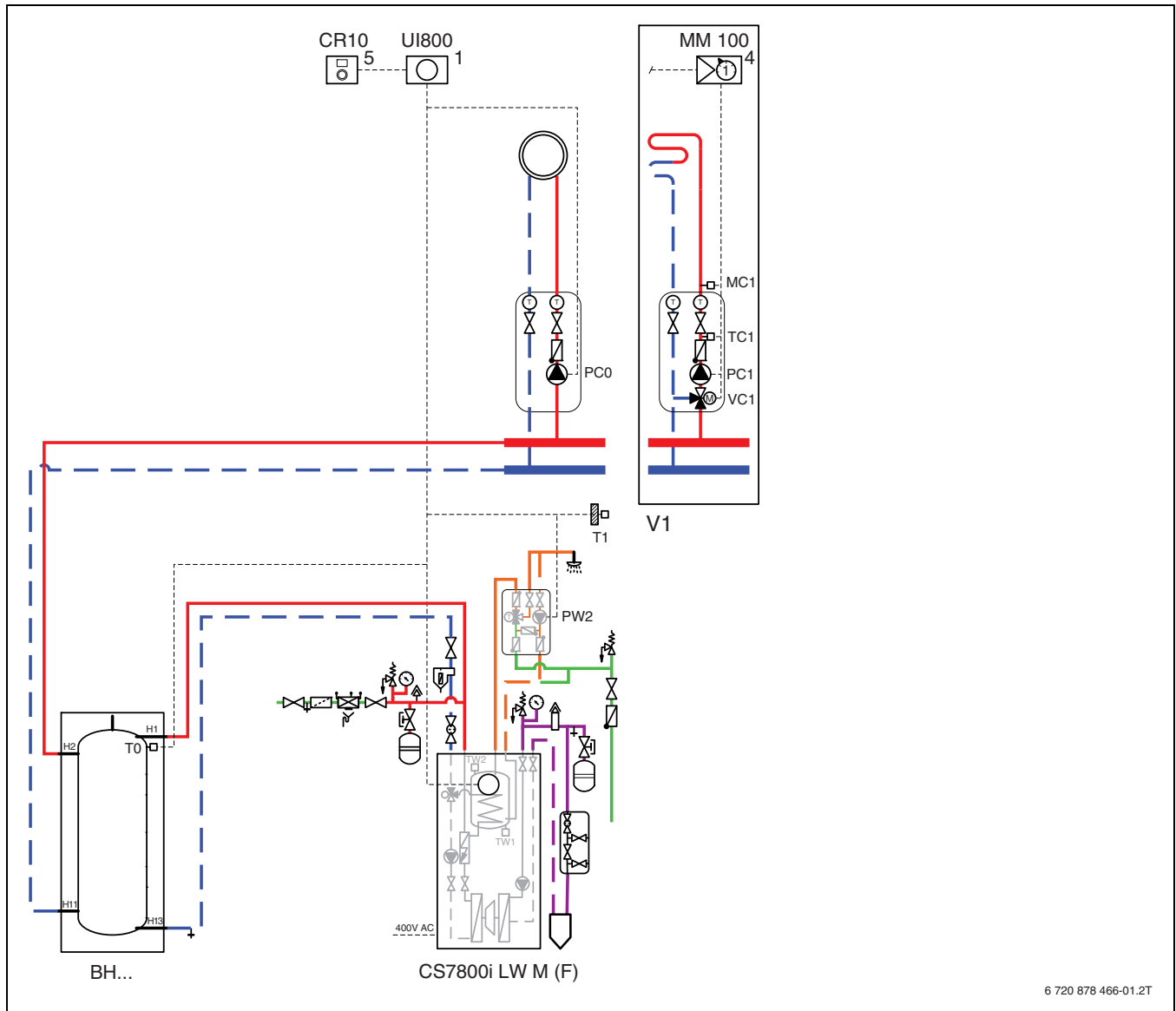
Bild 45 Parallele Pufferspeicher
