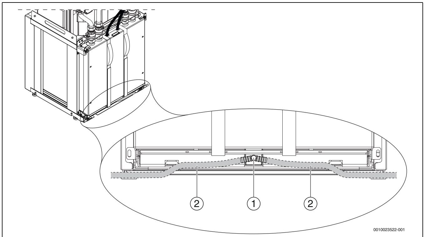
Bild 14 Anschluss des Ablassschlauches
