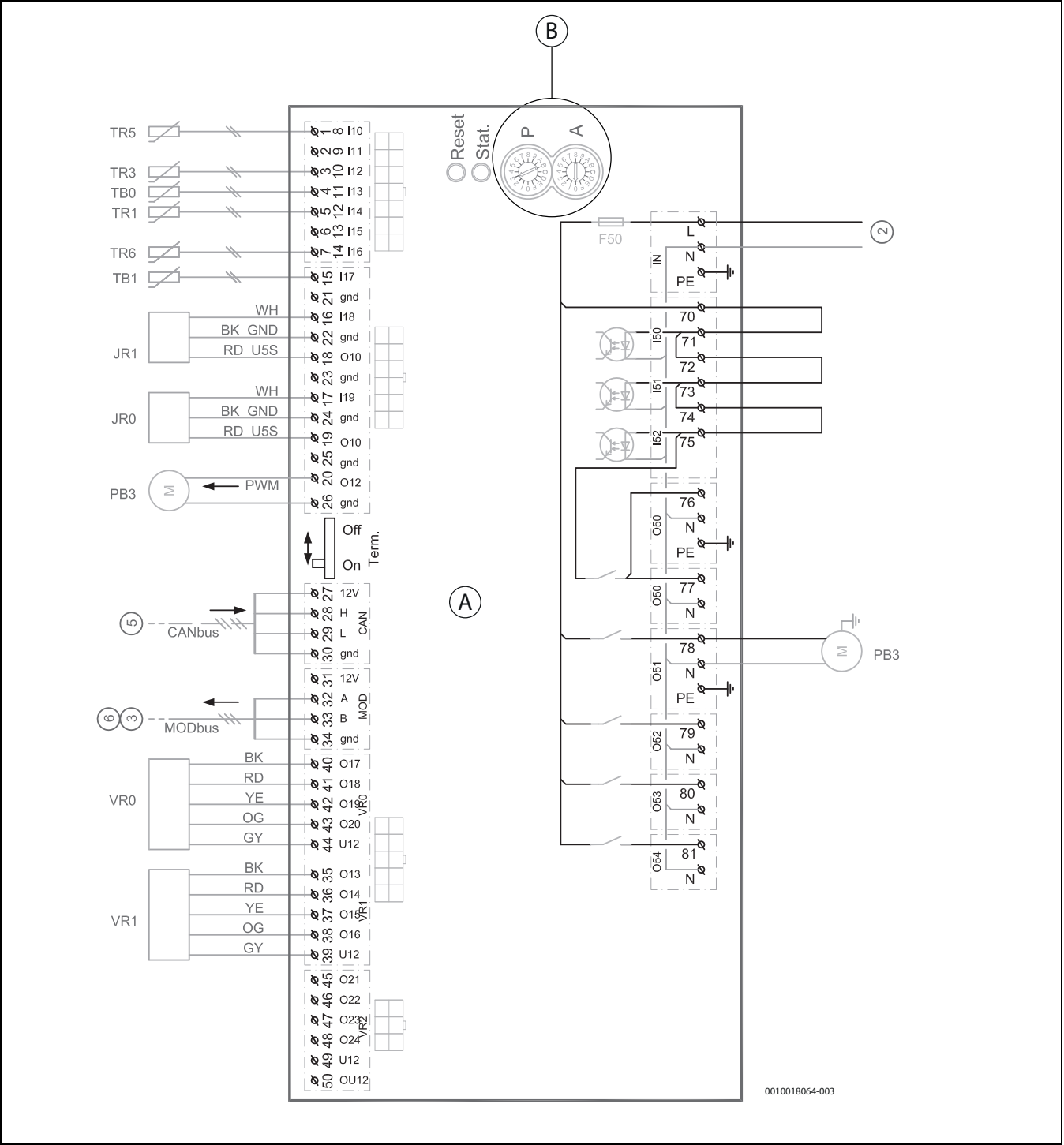
Bild 55 Schaltplan I/O-Modul
