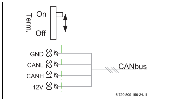
Bild 18 CAN-BUS-Terminierung
