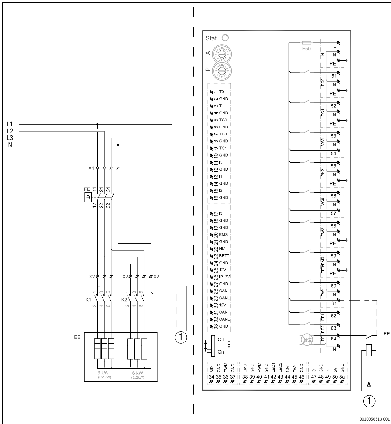
Bild 51 Verdrahtung des zusätzlichen Relais
