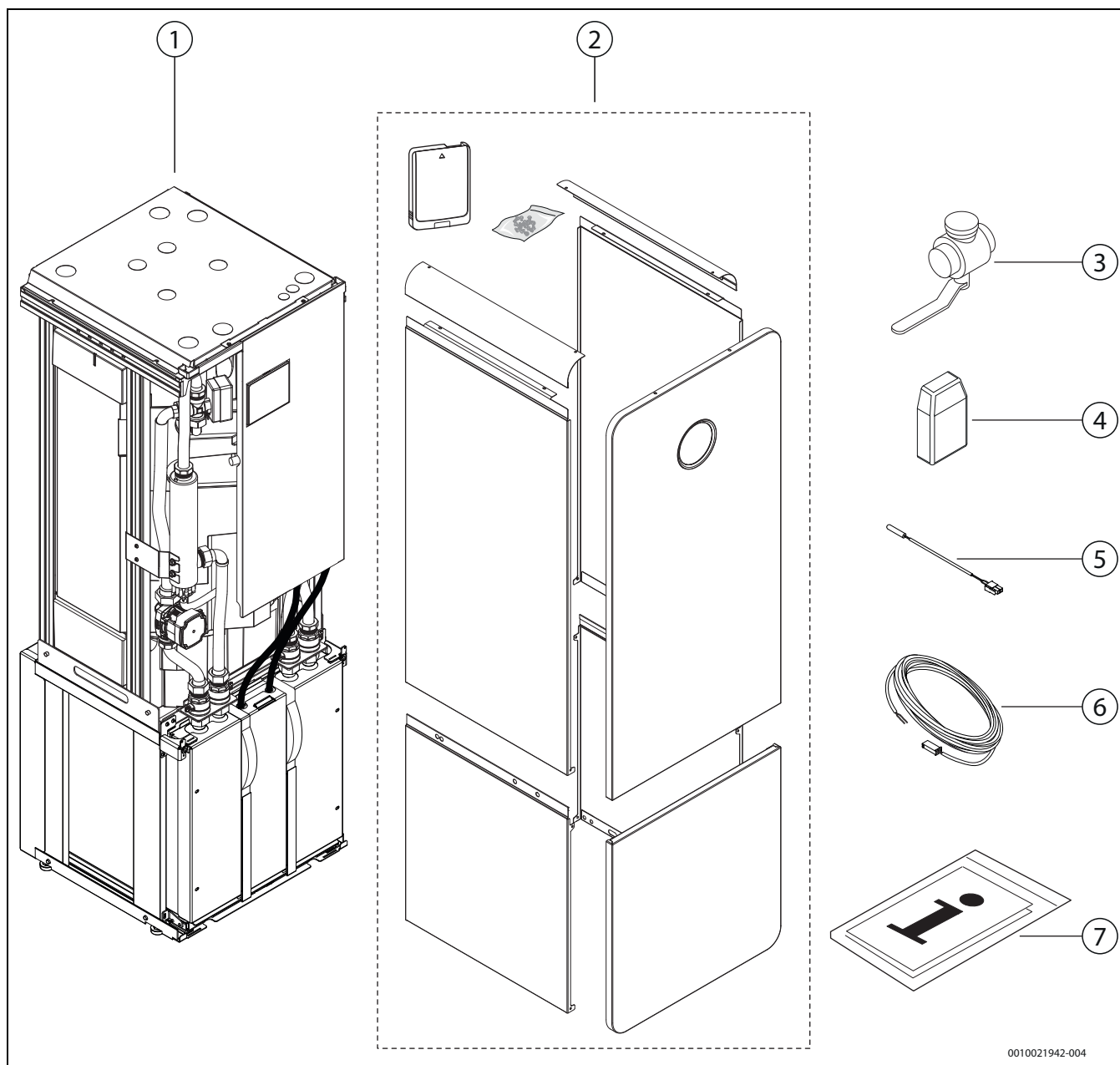
Bild 2 Lieferumfang
