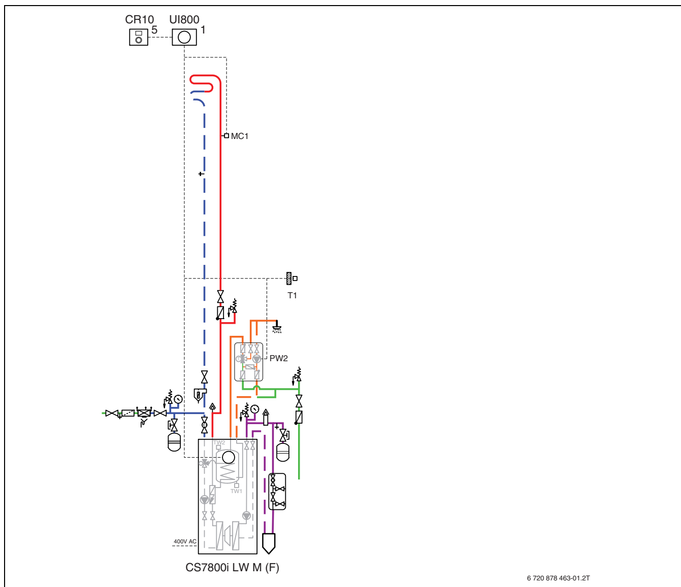
Bild 44 Standard
