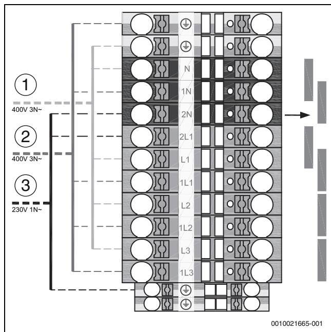
Bild 50 Spannungsversorgung EVU 2/EVU 3 mit drei Versorgungsleitungen (12 kW, 16 kW)
