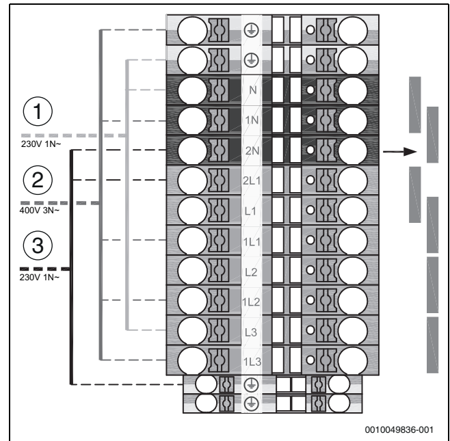
Bild 49 Spannungsversorgung EVU 2/EVU 3 mit drei Versorgungsleitungen (6 kW, 8 kW)
