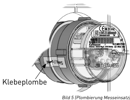
Bild 5 (Plombierung Messeinsatz)
