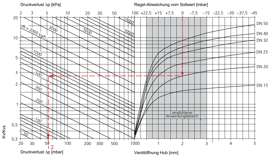
Diagramm TA-Multi mit Differenzdruckregler DN 15 (1/2") bis DN 50 (2")
