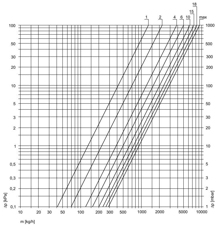
Voreinstellung mit Voreinstell- und Absperrhandrad
