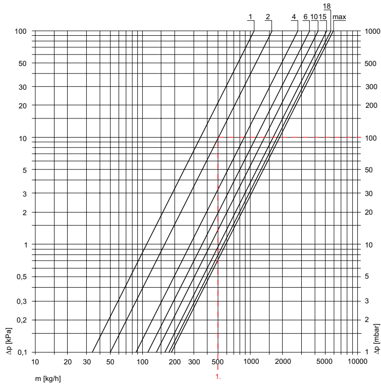
Voreinstellung mit Voreinstell- und Absperrhandrad
