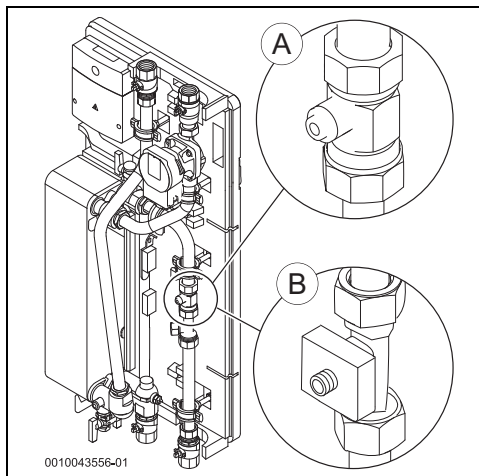
Fig. 1 Individuazione del flussostato/misuratore di portata (A = montato con il modulo NF \geq 27.07; B = montato con il modulo NF < 27.07)
