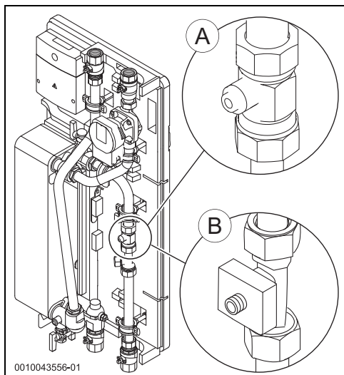
Rys. 1 Określanie czujnika natężenia przepływu (A = zamontowany z modułem NF ≥ 27.07; B = zamontowany z modułem NF < 27.07)
