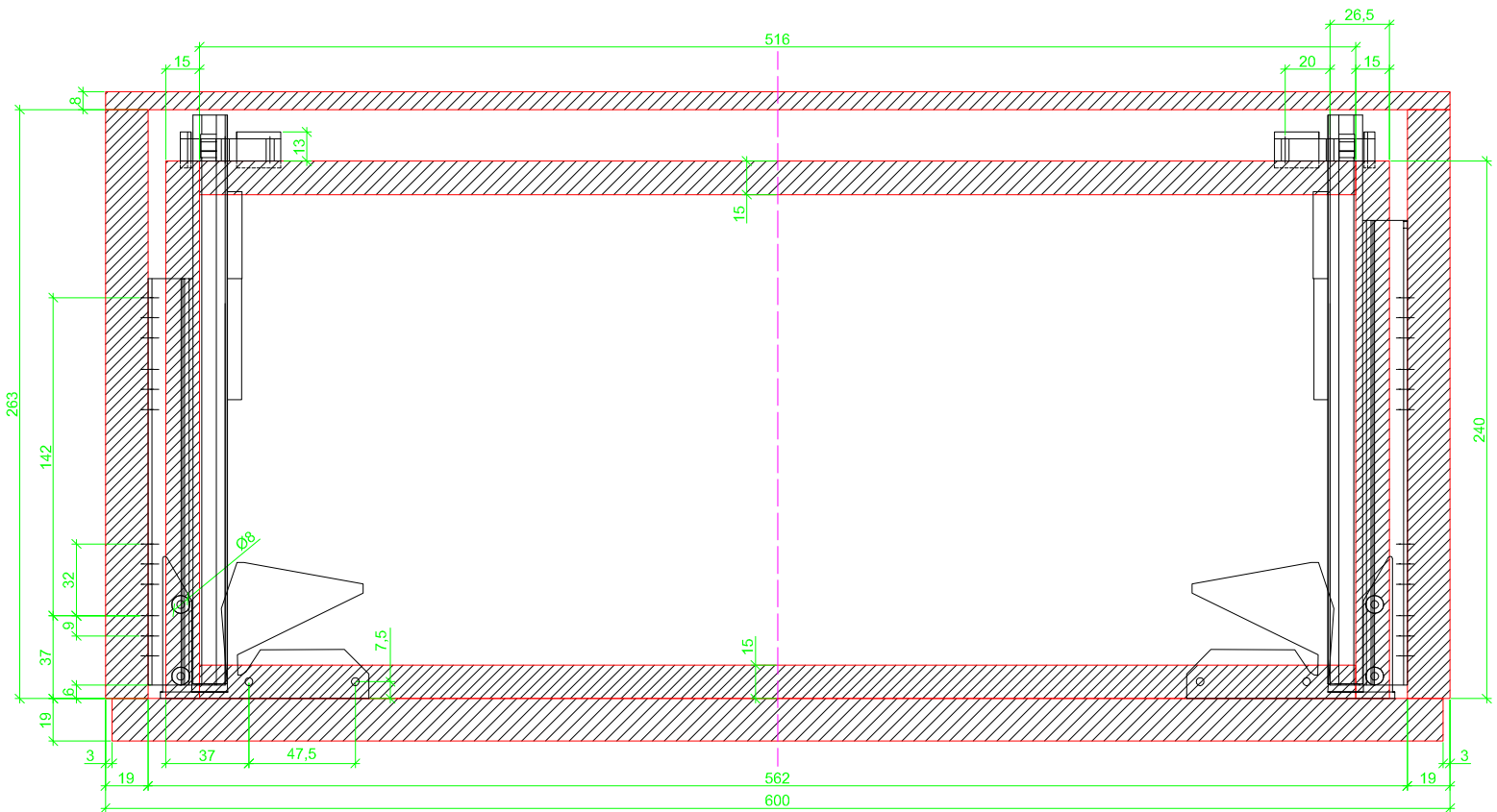
Drawer side on top of drawer bottom with Plug/ Seitenzarge auf Schubkastenboden mit Aufsteckhalter
