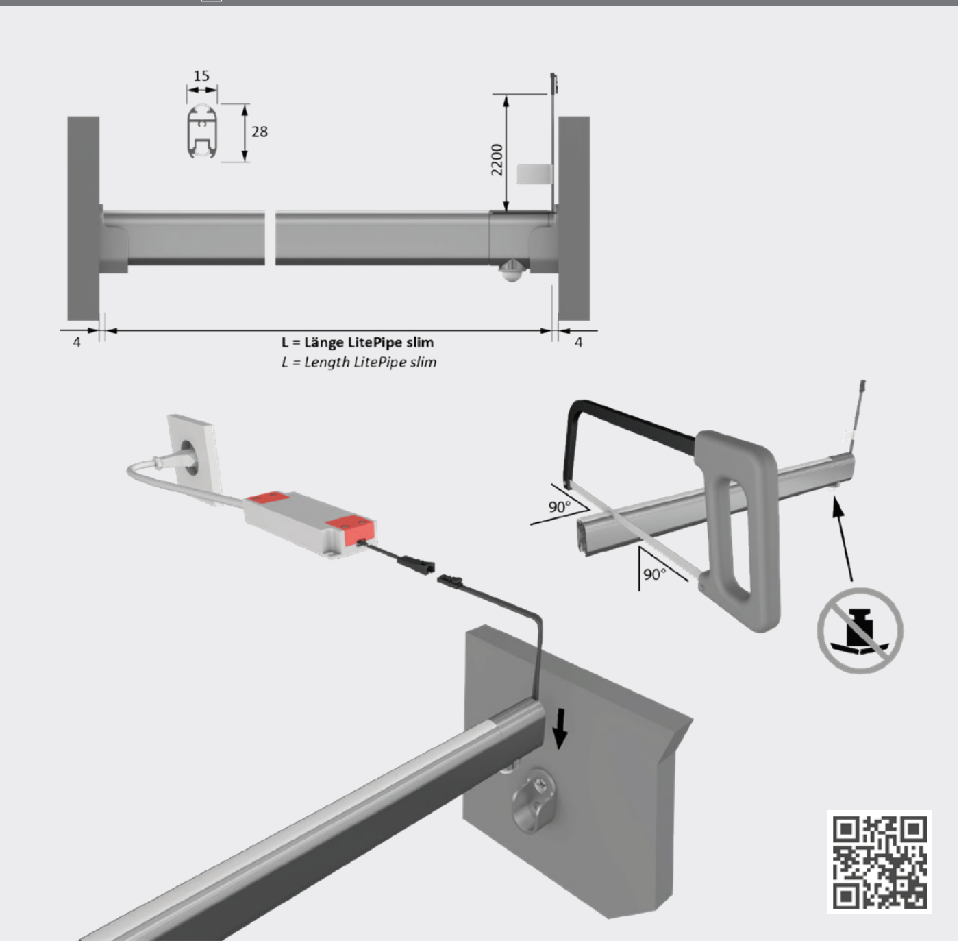
Montagezeichnung Individuell kürzbar
