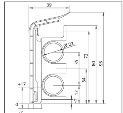
Abb. 2: Skizze Abmessungen HZ-SLF mit HZ-Schelle Artikel 2150 (nach der Rohrverlegung)
