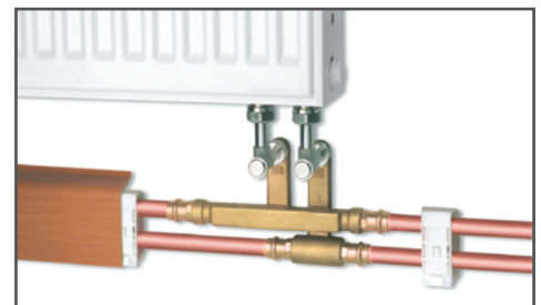
Abb. 10: HZ-Heizkörperanschluss
