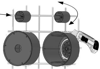
Bild 1 (Abtrennen Blistereinputzhaube)
