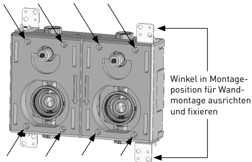
Bild 8 (Wandinstallation)
