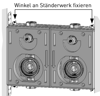
Bild 7 (Vorwandinstallation)
