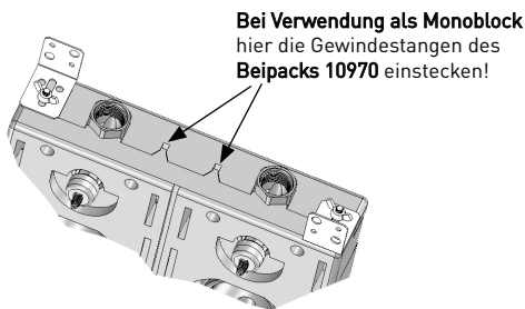
Bild 10 (Monoblock)
