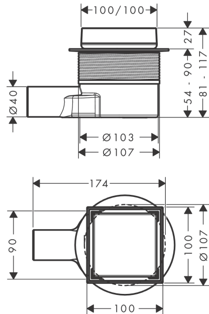
Maßzeichnung
