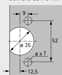
Bohrbild 52 x 9 mm
