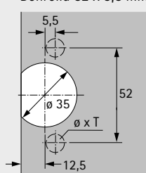
Bohrbild 52 x 5,5 mm
