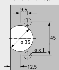
Bohrbild 45 x 9,5 mm
