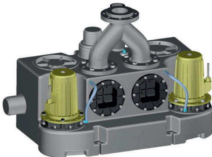
SANICUBIC 2 VX KB 1.1 und 1.5 mit innenliegenden Rückschlagklappen
