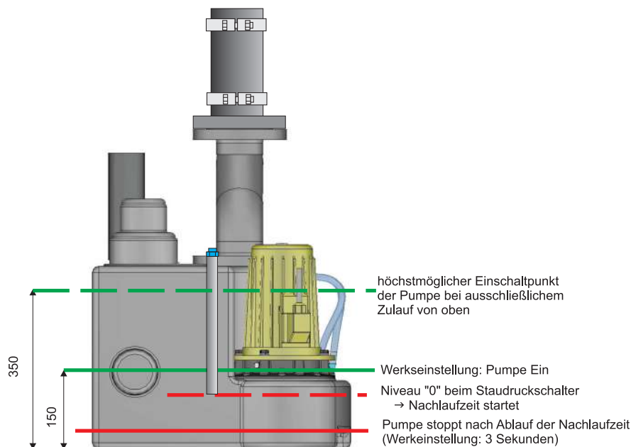
Funktionsprinzip der Niveausteuering
