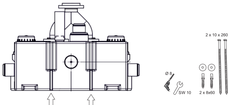
Befestigungspunkte hinten
