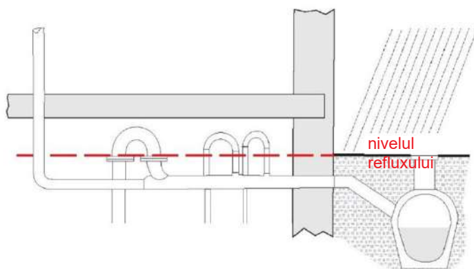
Exemplu de buclă de refluxare
