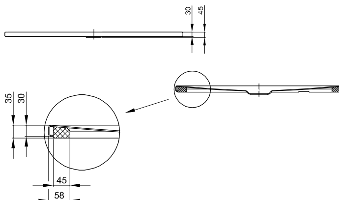
Darstellung mit vormontiertem Minimum-Wannenträger (T1).
