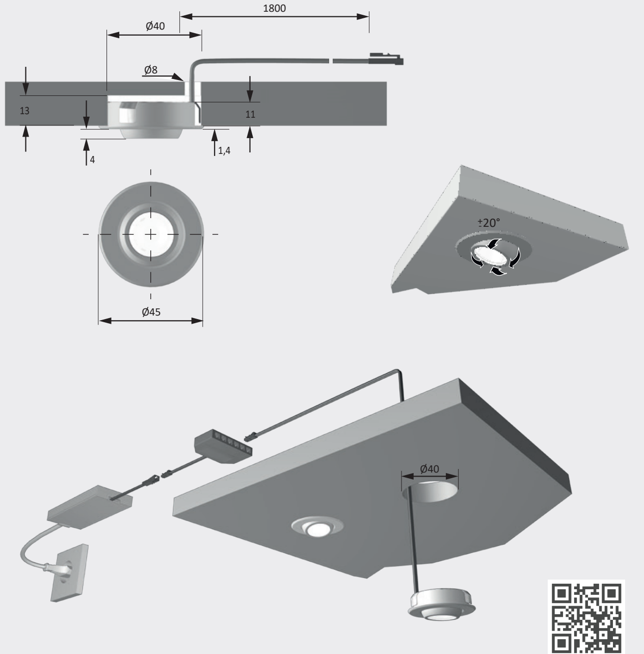
Montagezeichnung
