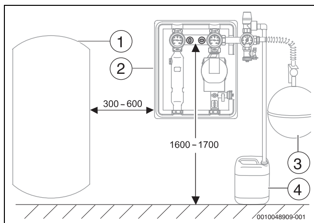
Bild 19 Empfohlene Aufstellung (Maße in mm)
