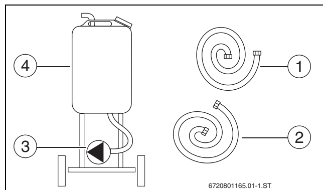
Bild 26 Bestandteile einer Befülleinrichtung
