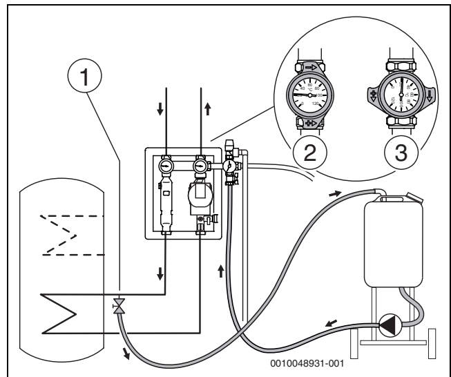
Bild 28 Spülen oberhalb der Solarstation
