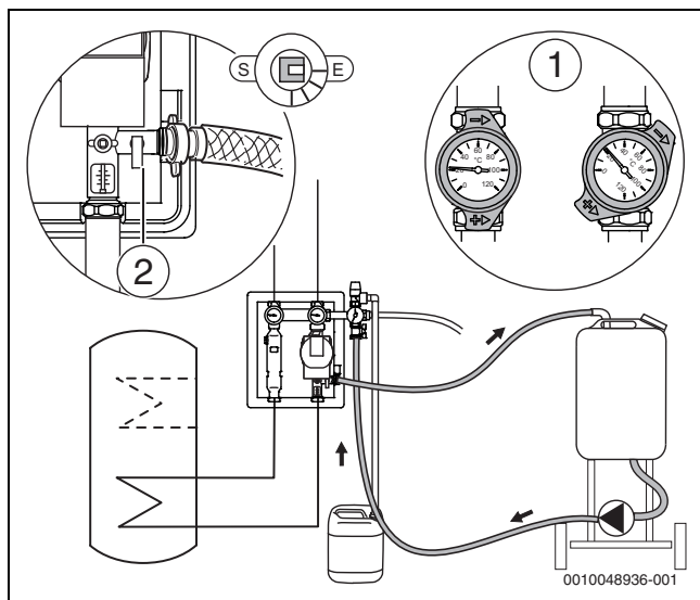
Bild 36 Spülen des Standardsystems
