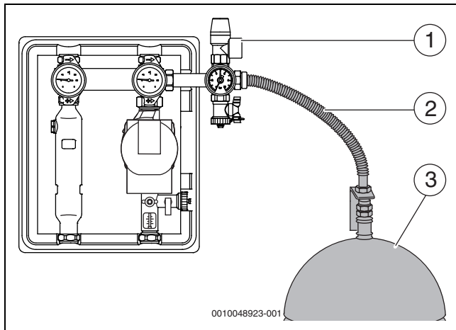
Bild 23 Montage des Ausdehnungsgefäßes
