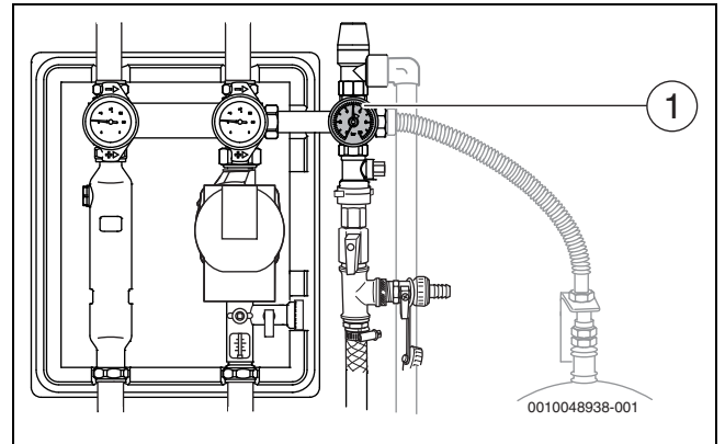
Bild 44 Manometeranzeige prüfen
