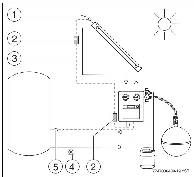
Bild 25 Temperaturfühler an Solarstation mit integriertem Regler
