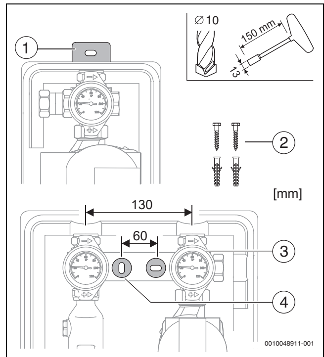
Bild 20 Montage der Station
