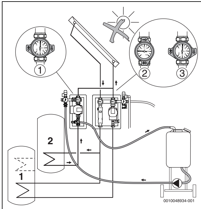
Bild 34 Spülen von Speicher 2
