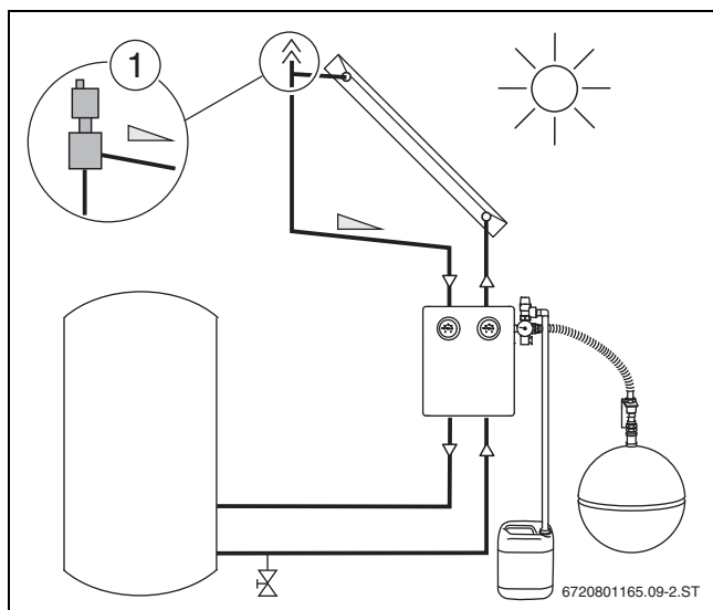
Bild 16 Position des automatischen Entlüfters
