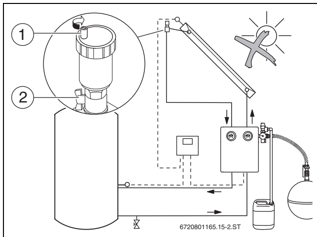
Bild 45 Entlüfter und Kugelhahn schließen
