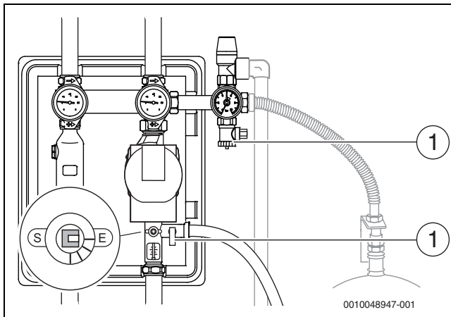
Bild 43 Befüllung über Füll- und Entleerhahn
