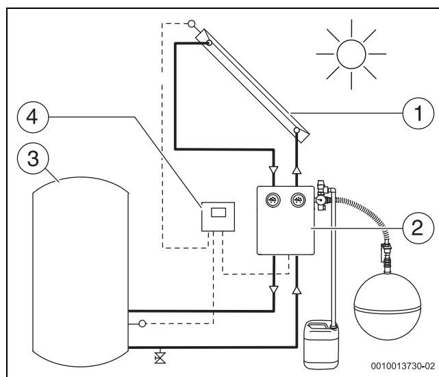
Bild 8 Beispielhafte Darstellung einer Solaranlage
