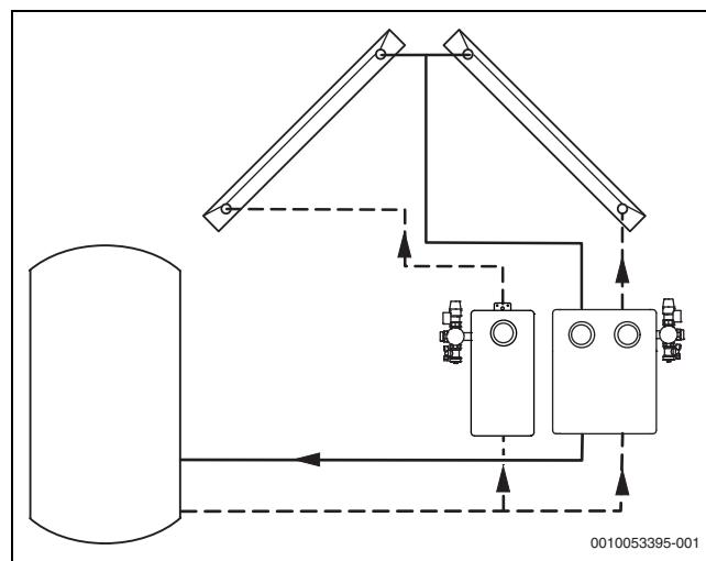
Bild 5 2 Kollektorfelder (Ost/West) mit 1- und 2-Strang-Solarstation
