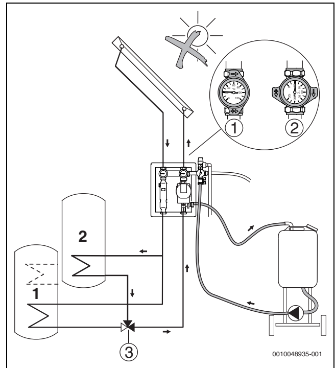
Bild 35 Spülen von Speicher 2
