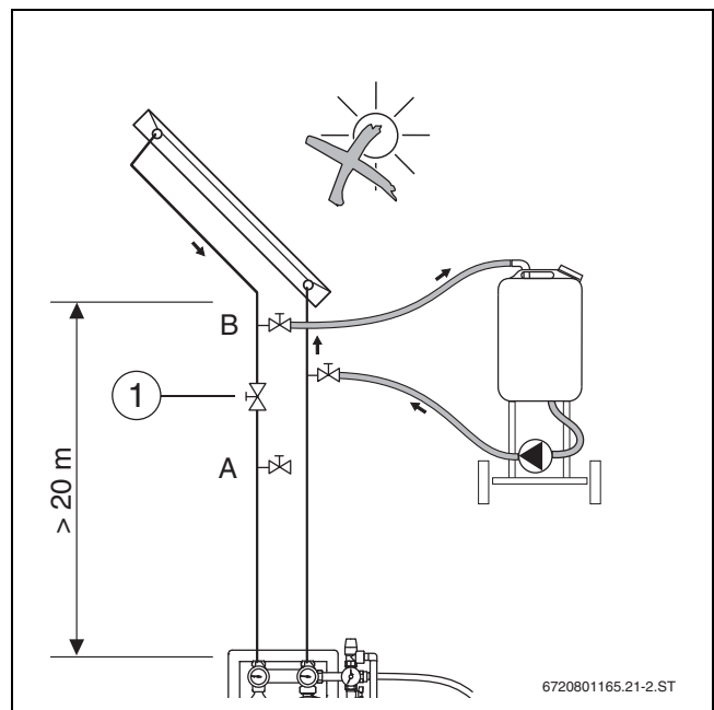
Bild 29 Oberen Anlagenteil spülen
