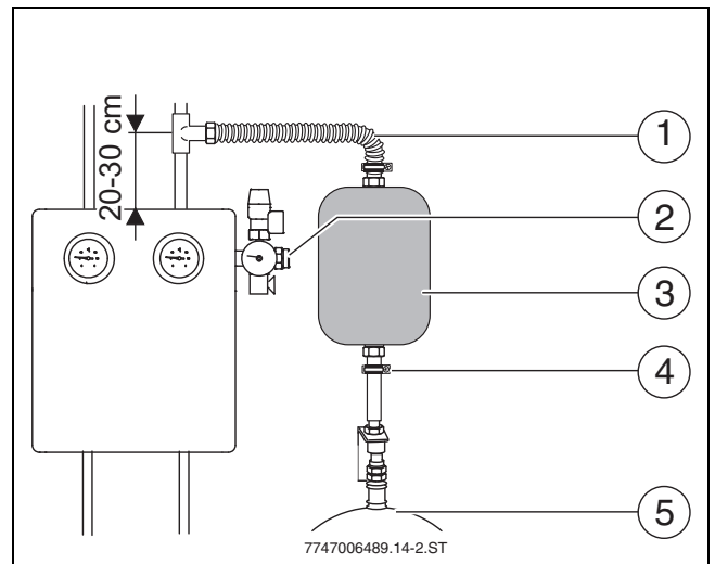
Bild 22 Montage des Vorschaltgefäßes
