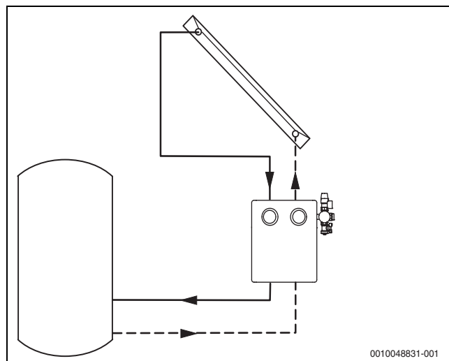
Bild 4 Standardsystem mit 2-Strang-Solarstation
