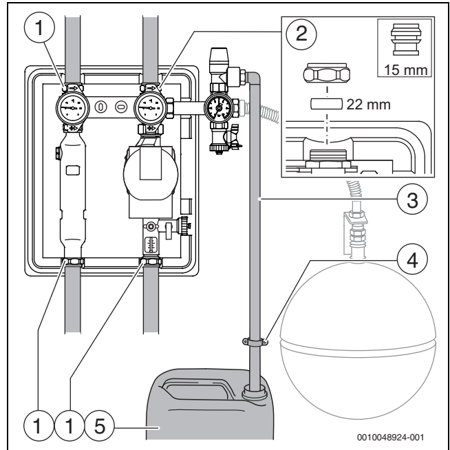
Bild 24 Anschluss an die Solarstation
