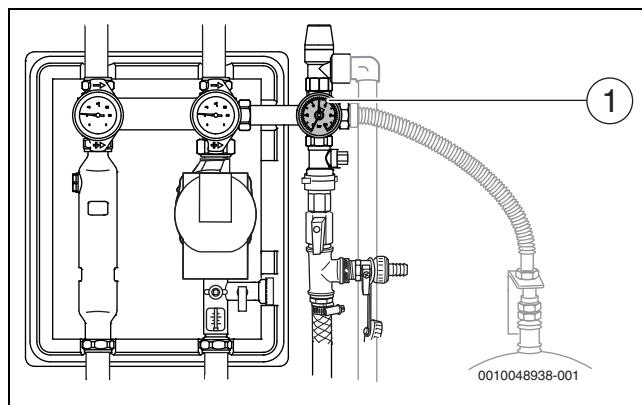
Bild 38 Manometeranzeige prüfen
