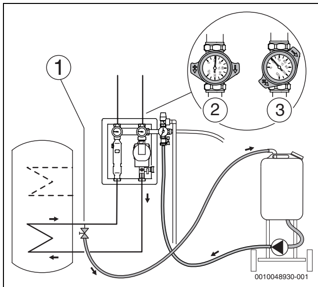
Bild 27 Spülen unterhalb der Solarstation
