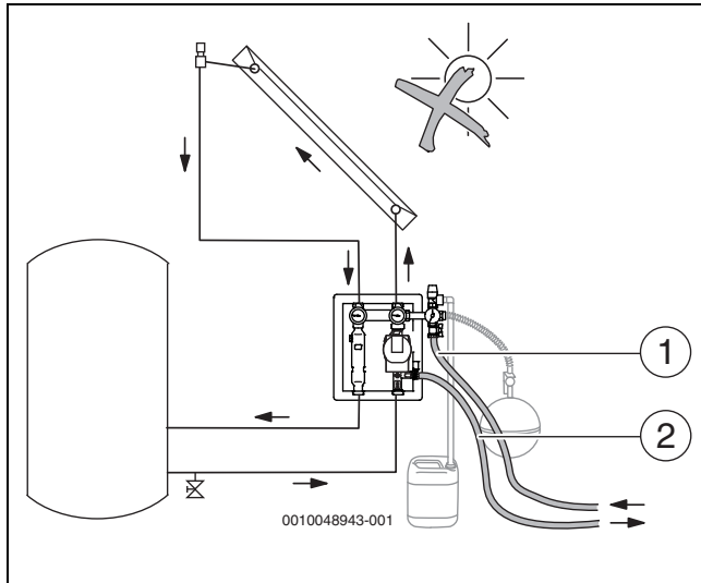
Bild 39 Solarstation mit Kugelhähnen und Schwerkraftbremsen in den Thermometern
