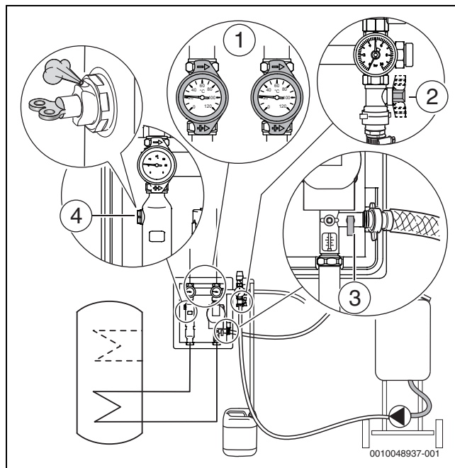
Bild 37 Füll- und Entleerhähne schließen und öffnen
