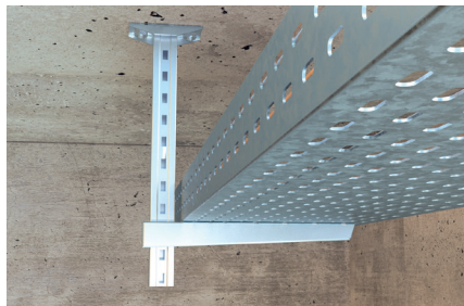
Kabeltrassen
