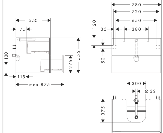
Maßzeichnung
