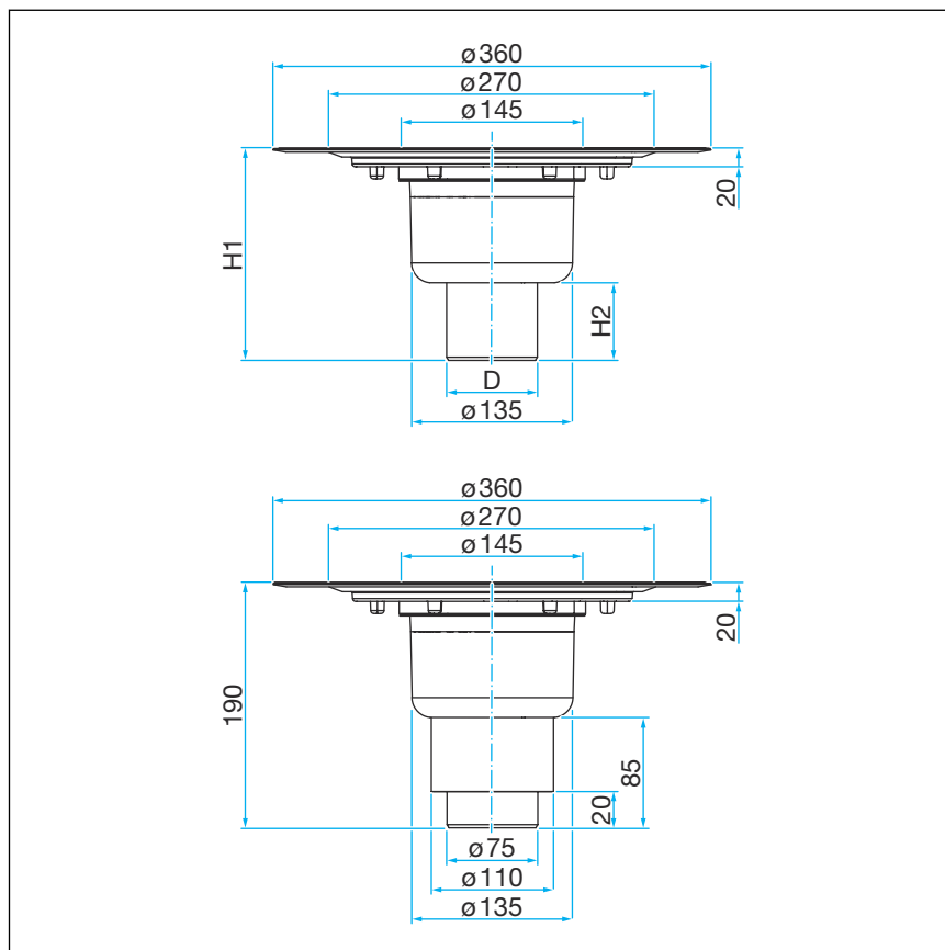
Abb. 5: Maßzeichnung Modell 4951.15
