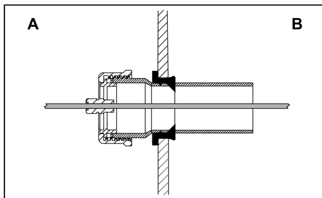
(A) Lato interno del serbatoio con terminale avvitabile (B) Lato esterno del serbatoio con collegamento per il tubo per cavi
