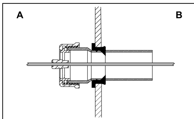
(A) Paroi intérieure de la cuve avec embout à visser (B) Paroi extérieure de la cuve avec raccord pour fourreau pour câbles
