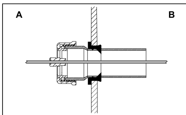
(A) Behälterinnenseite mit verschraubbarem Endstück
