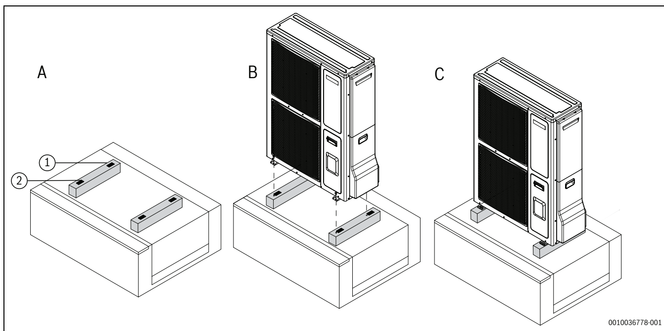
Bild 7 Bodenstehende Außeneinheit
