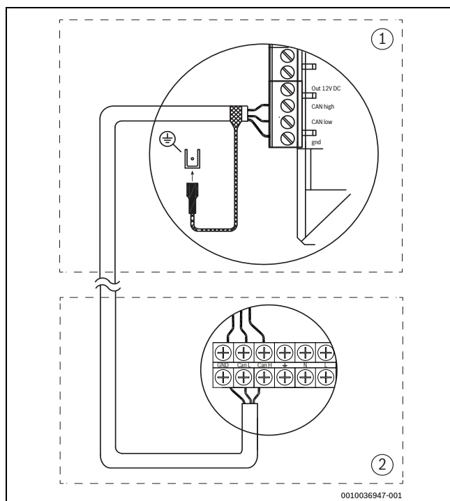
Bild 18 CAN-BUS-Verbindung
