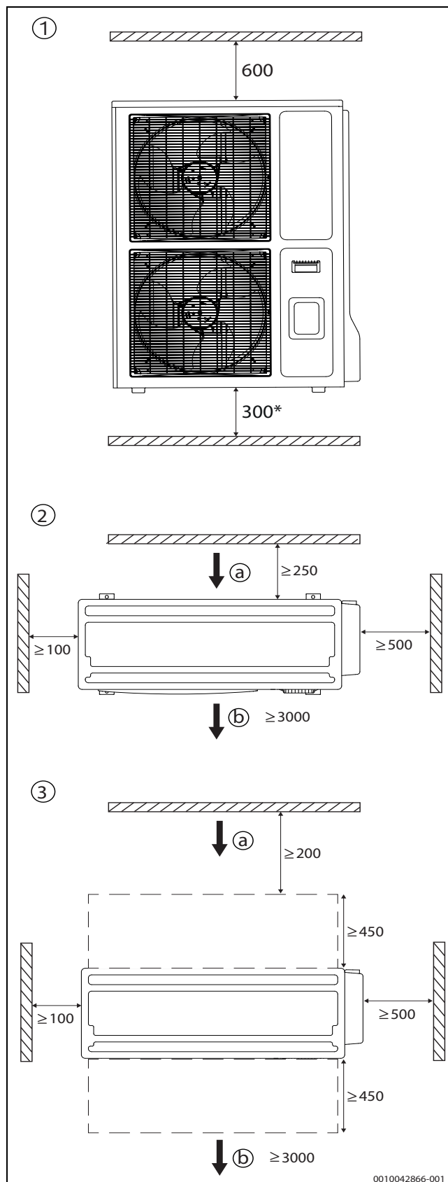
Bild 3 Mindestabstände (mm)
