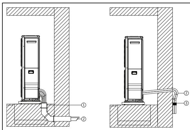
Bild 15 Anschluss der Außen- an die Inneneinheit
